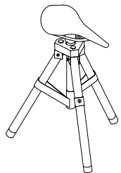
banco_bike peça central em madeira escala 1:1
